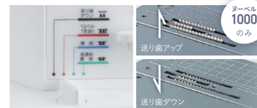
4段階の送り歯高さ調節 ブラザーオリジナル
